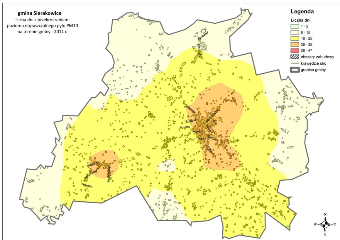
Rysunek 3. Rozkład liczby dni z przekroczeniem dopuszczalnego stężenia 24-godzinnego dla pyłu PM10 na terenie Gminy Sierakowice w roku bazowym 2011 (źródło: opracowanie własne na podstawie POP dla strefy pomorskiej)
