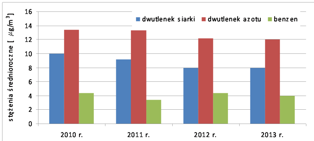
Rysunek 2. Poziomy stężeń średniorocznych dwutlenku siarki, dwutlenku azotu i benzenu w m. Sierakowice w latach 2010-2013 (Roczna ocena powietrza w województwie pomorskim. Raport za rok 2013 r. WIOŚ w Gdańsku)
