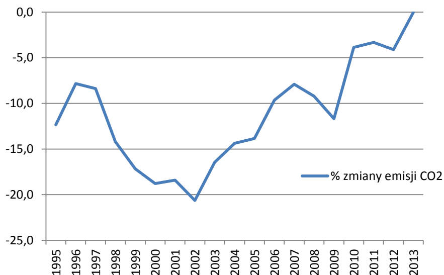
Rysunek 19. Zmiany emisji CO 2 w gminie Sierakowice w latach 1995 – 2013, w stosunku do roku bazowego 2013 [%] (źródło: opracowanie własne na podstawie danych GUS)
