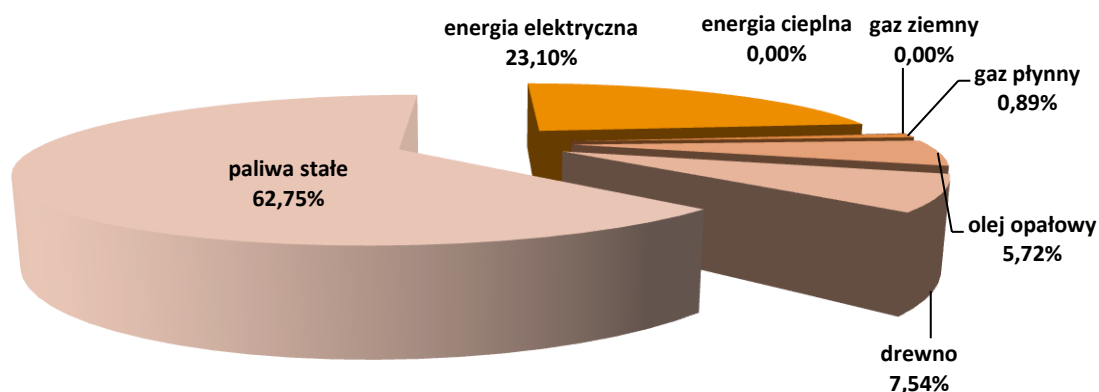
Rysunek 9. Struktura udziałów poszczególnych paliw oraz energii cieplnej i elektrycznej używanych w Gminie Sierakowice w emisji dwutlenku węgla 18
